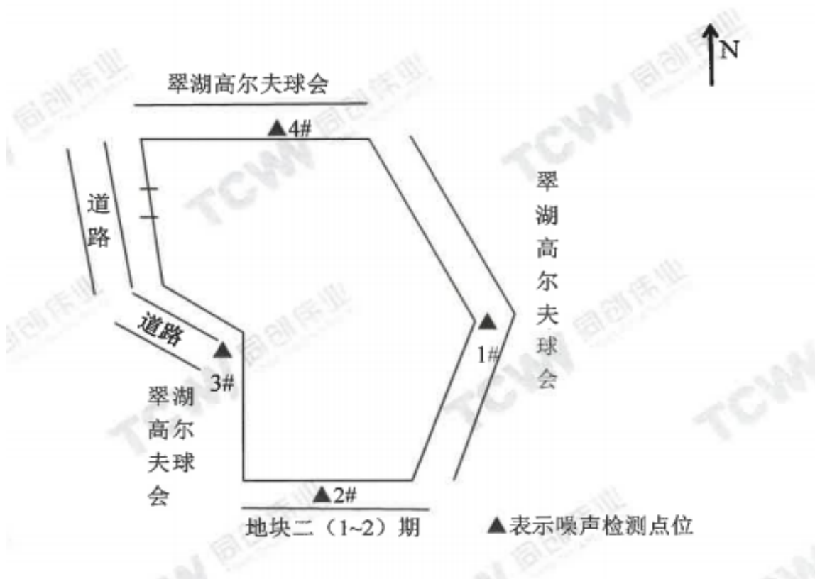
图 8.2-1 建设项目噪声监测点位平面示意图
